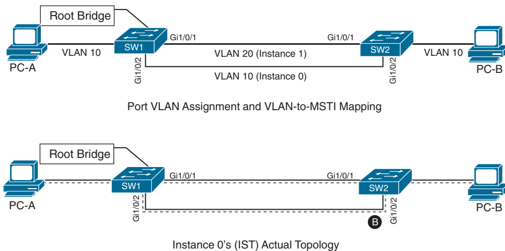
Figure 4-5 Understanding the IST Topology
