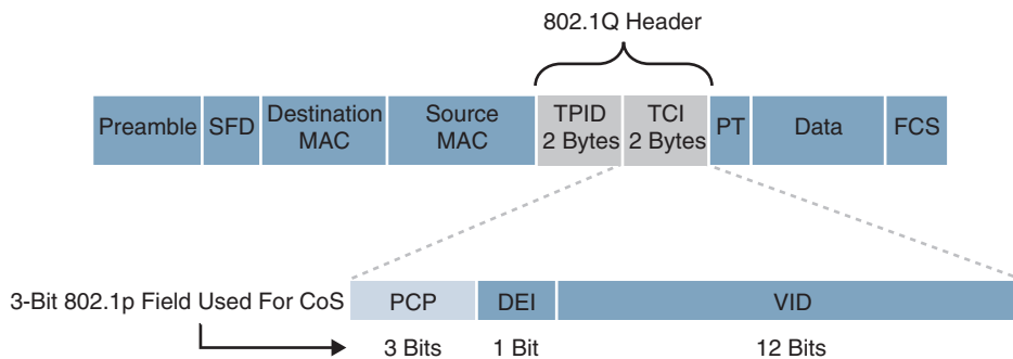
Figure 14-4 802.1Q Layer 2 QoS Using 802.1p CoS
