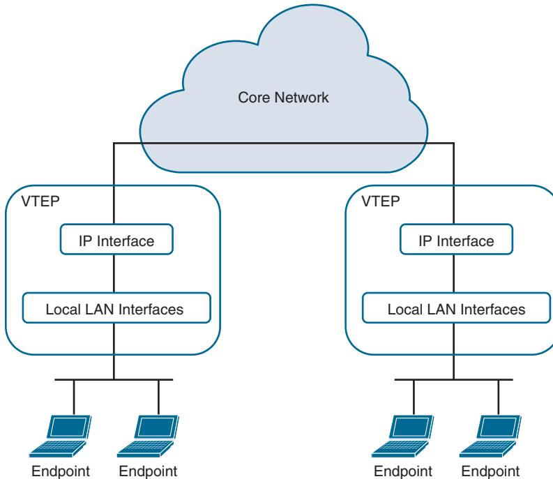
Figure 16-14 VXLAN VTEP
